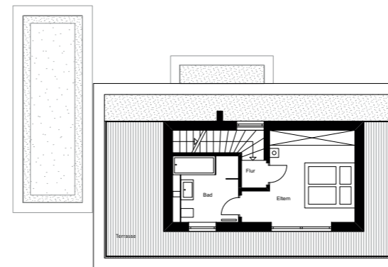
Dachgeschoss
